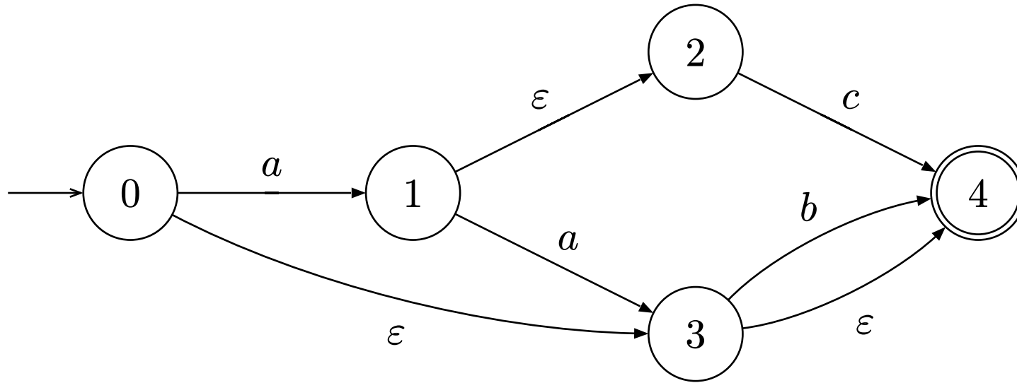
Fig. 1. – Automate à \varepsilon -transitions reconnaissant \{\varepsilon, b, ac, aa, aab\} .
